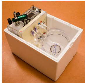
Foto van het prototype van de Organ Assist leverbox
